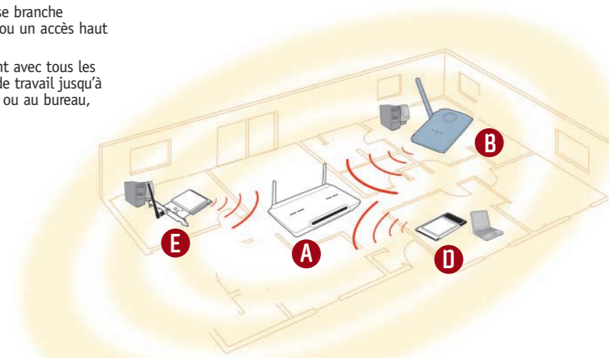
A Routeur câble/ADSL sans fil - F5D6231fr4 B Adaptateur réseau USB sans fil - F5D6050f C Point d'accès réseau sans fil - F5D6130f (voir panneau latéral) D Carte réseau sans fil pour ordinateurs portables - F5D6020f E Carte réseau sans fil PCI - F5D6001fr
